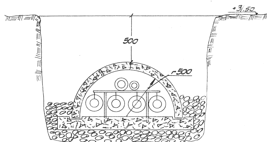
Snitt I-I Skala 1:20
